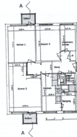
PLATTEGROND NIEUWE TOESTAND SCHAAL 1:100
