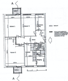
PLATTEGROND NIEUWE TOESTAND SCHAAAL 1:100
