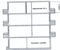
DOORSNED E AA - NIEUWE TOESTAND SCHAAL 1:100
