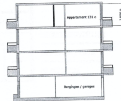
DOORSNED E AA - NIEUWE TOESTAND SCHAAL 1:100
